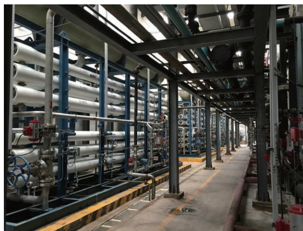
煤化工浓盐水处理装置
